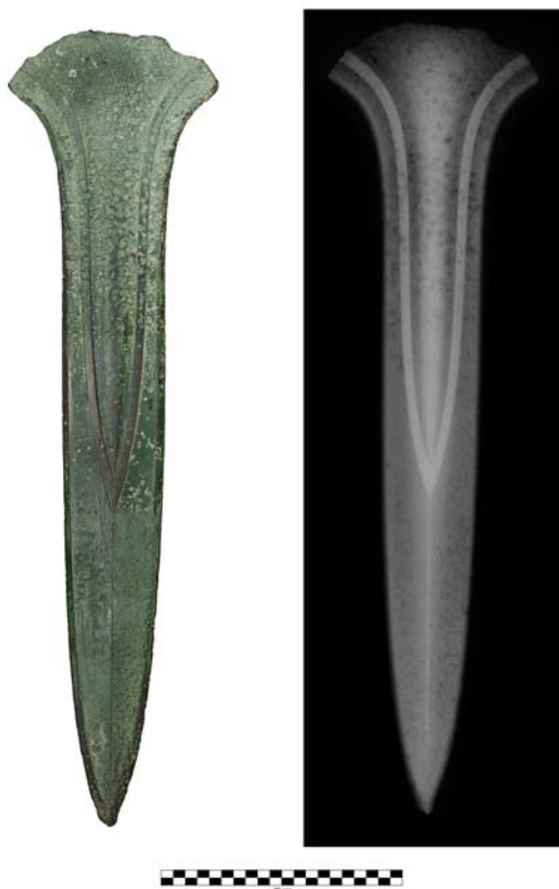
Fig. 7 - Radiographie de l'épée de Plougrescant. Crédits : C2RMF.
