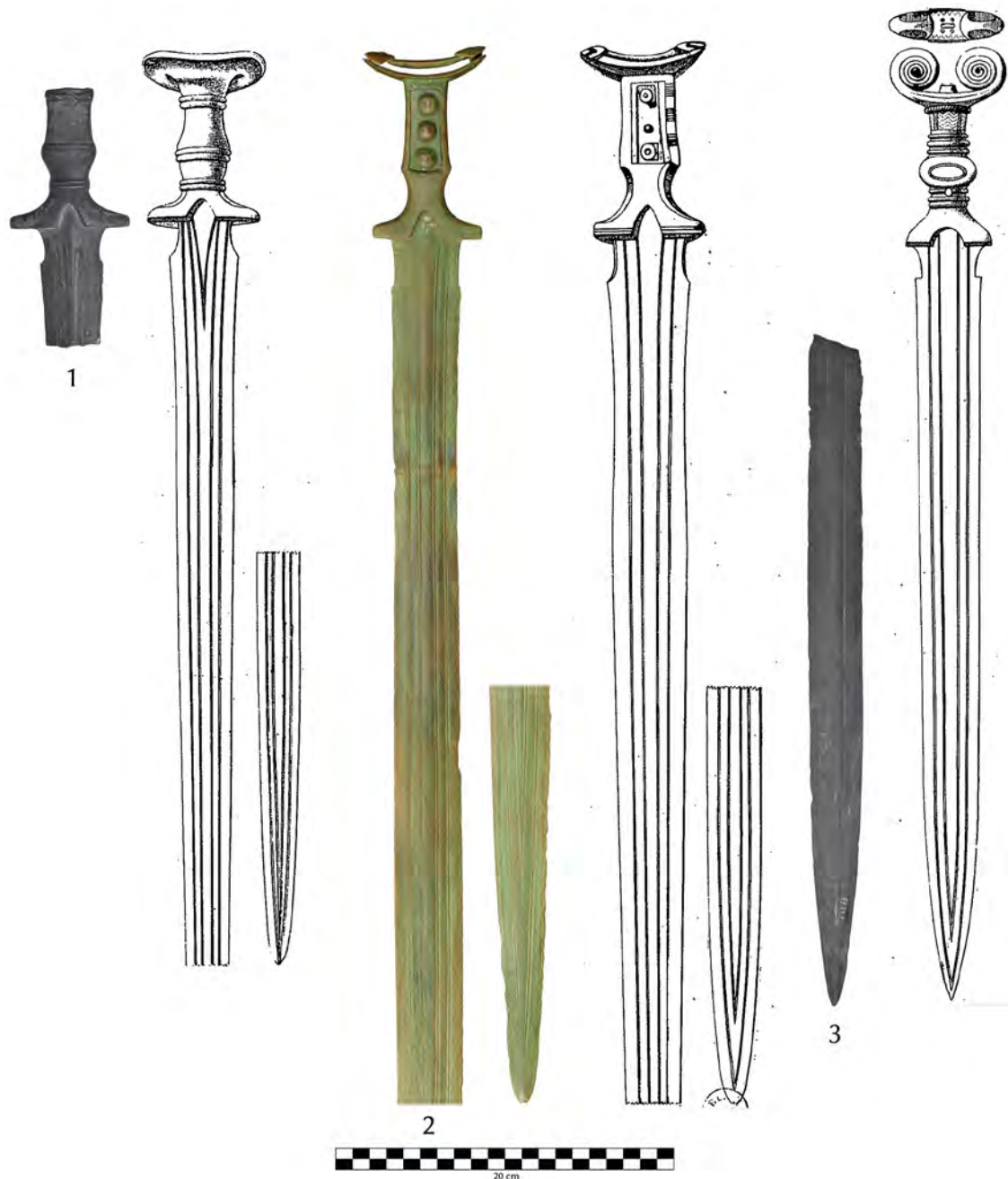
Fig. 3 : Comparaison entre les épées d'Aliès telles que représentées en 1872 (d'après Rames 1872) et leur état de conservation actuel. 1. Musée Bargoin, Clermont-Ferrand, n° 57.81.1. 2. British Museum, n° 1890,5-19.1. 3. Musée Bargoin, Clermont-Ferrand, n° 57.84.1
