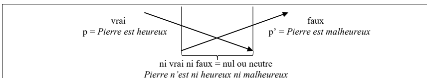
Figure 3 : Opérateurs logico-linguistiques
