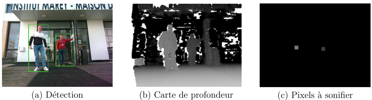
Figure 4.7: Vue d'ensemble de la méthode : d'abord un CNN estime les positions des personnes à partir de l'image couleur (a), ensuite la distance à l'utilisateur est extraite de la carte de profondeur (b) pour générer le pixel à sonifier (c).
